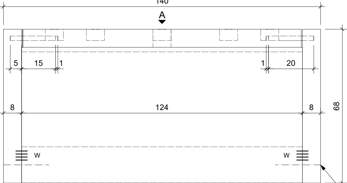
Vorderansicht C
