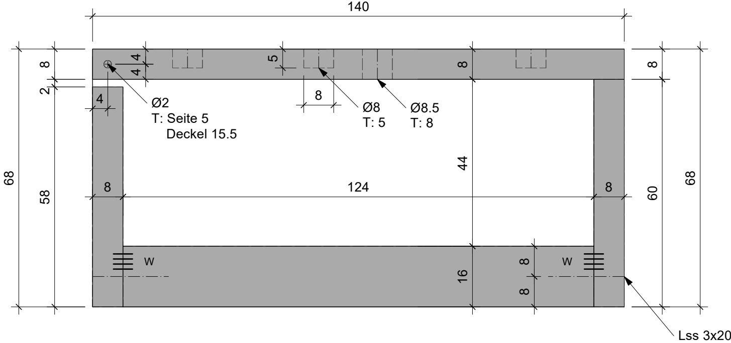
B-B
