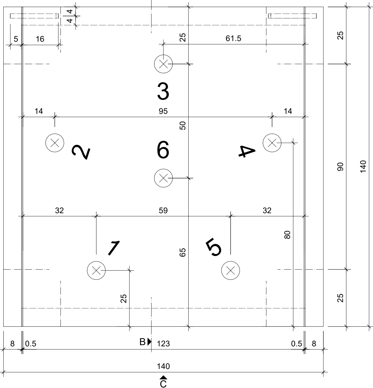
Draufsicht A
