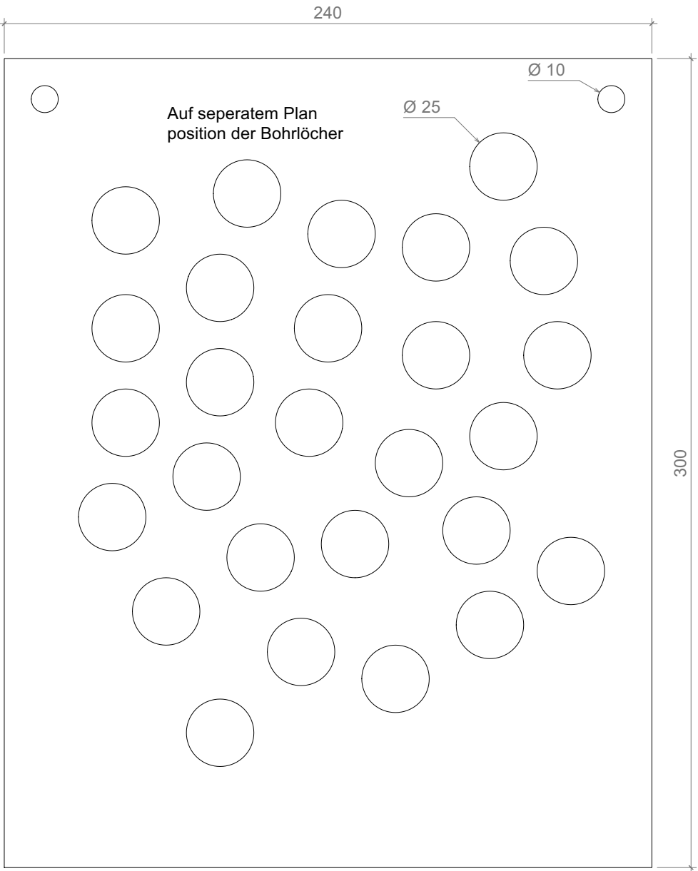
Ansicht C Spielfeld
