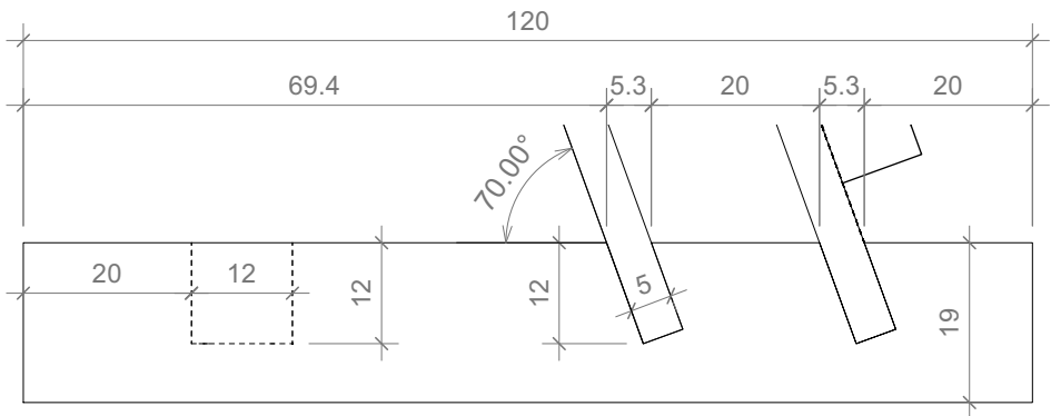
Detail Seitenansicht B
