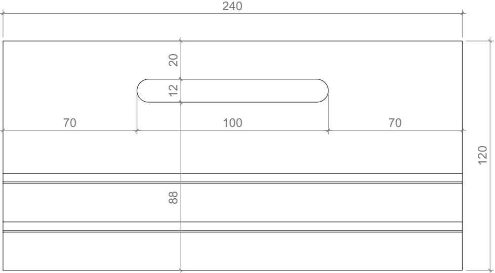
Draufsicht A Grundplatte
