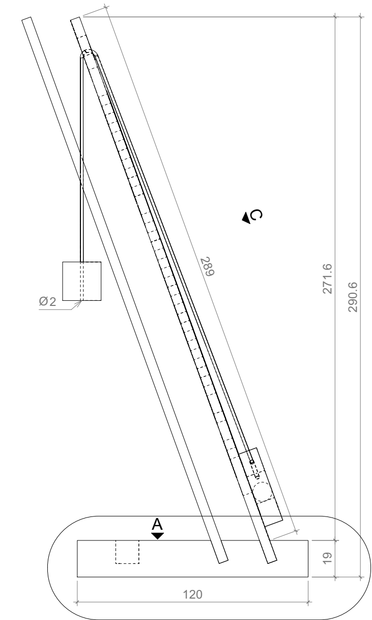
Seitenansicht B (ganzes Spiel)
